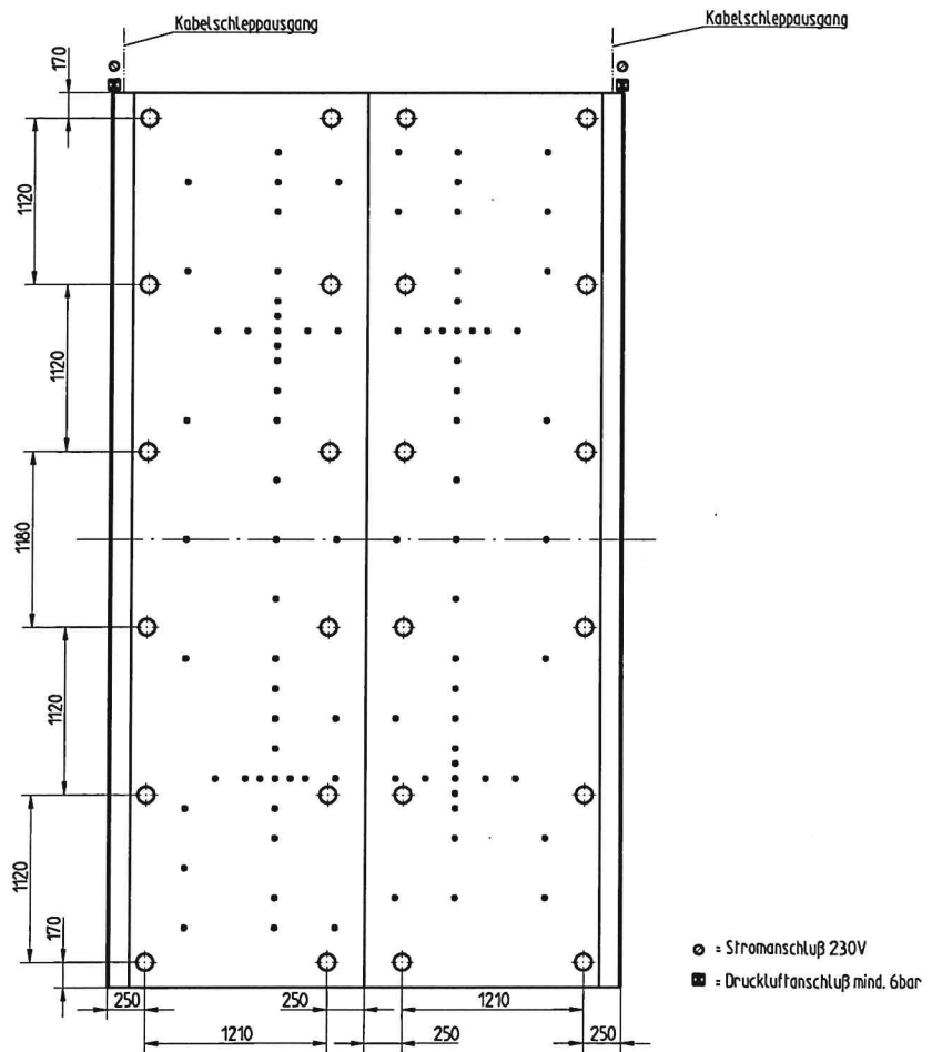
Draufsicht ohne Meßmaschine gezeichnet
